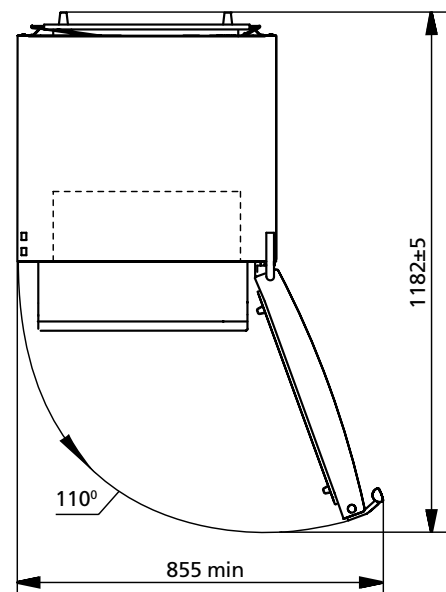
Малюнок 2 – Холодильник (вид зверху)
