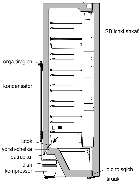
8-rasm. SBdan erigan suvni oqozish sxemasi
