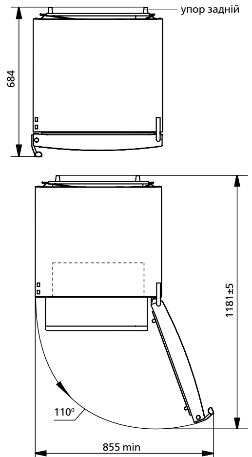
Малюнок 2 – Холодильник (вид зверху)
